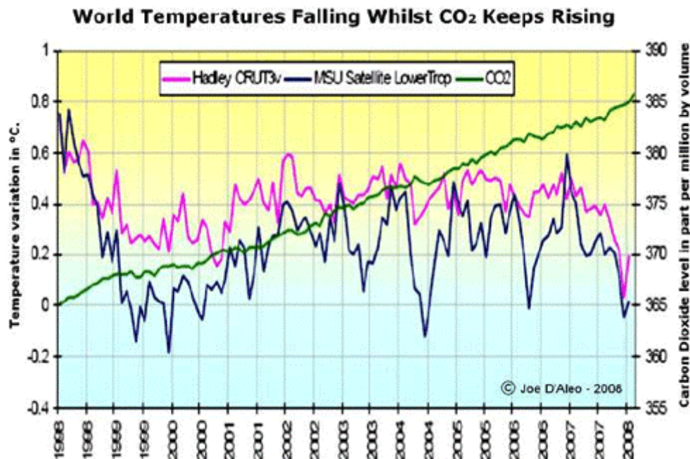
Abb. 2 Temperatur nach CRU (England) in violett, Temperatur nach Satellitenmessungen MSU in blau, CO 2 , Mauna Loa in grün. Quelle: Joe D'Aleo 2008; http://www.climate-science.org.nz/images/PDFs/ipcc_letter_14april08.pdf
