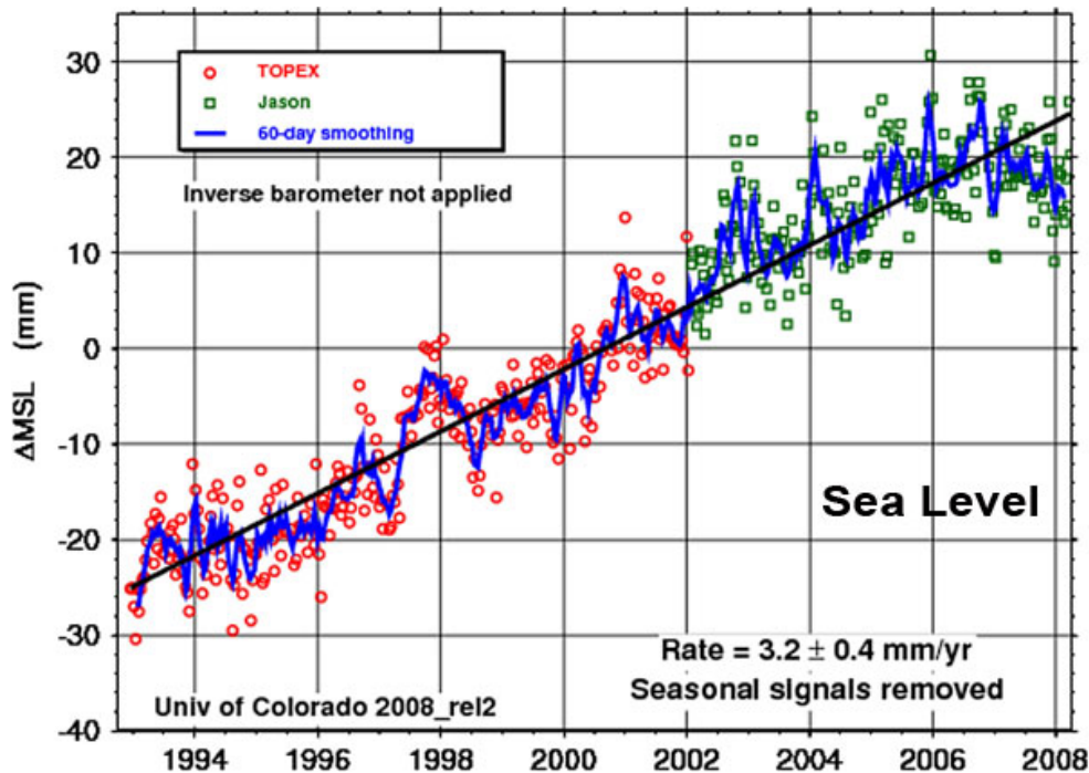
Abb. 2 Gemessene Meeresspiegel durch die Satelliten Topex und Jason Quelle: http://icecap.us/images/uploads/SeaLevel_TOPEX.jpg ; http://topex-www.jpl.nasa.gov/
